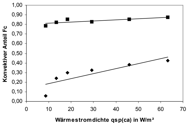
Bild 4 Konvektionsanteil
