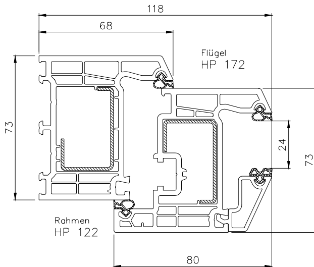
Bild 1 Foto/Zeichnung Querschnitt
