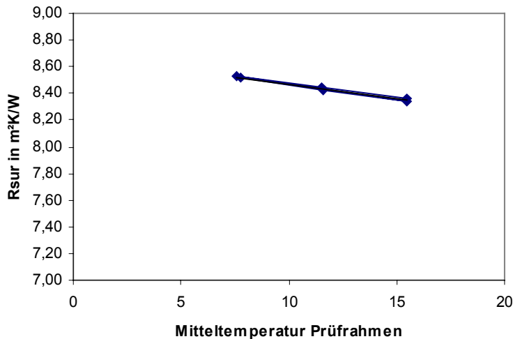
Bild 2 Wärmedurchlasswiderstand Umfassungrahmen
