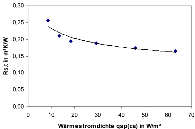
Bild 3 Gesamtwärmeübergangswiderstand
